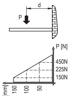
DIAGRAMMA DI CARICO LOADING CAPACITY DIAGRAM
